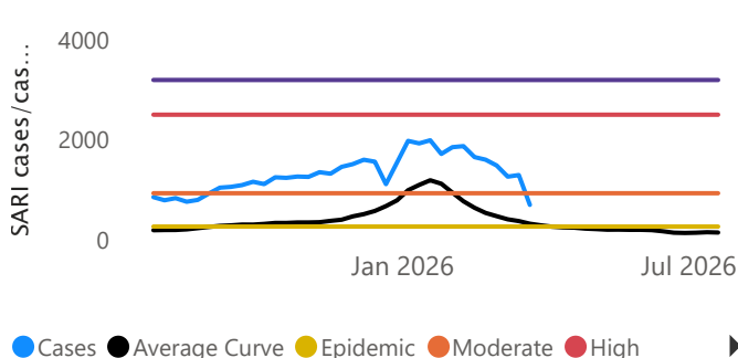
No. new SARI cases by EW/N° de casos IRAG nuevos por SE
