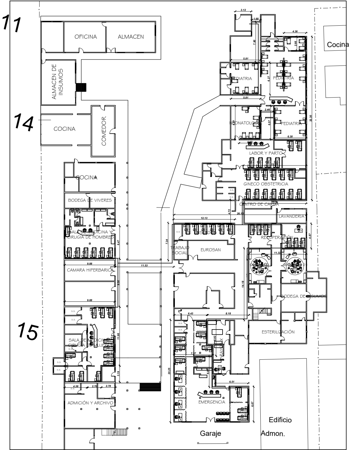
PLANTA DE RED DE OXIGENO INSTALACIÓN DE RED DE OXIGENO DEL HOSPITAL PUERTO LEMPIRA ARP USAID
